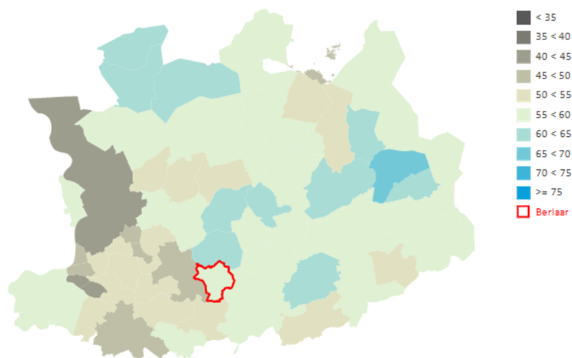
FIGUUR 2: Responsgraad (%) per gemeente. Antwerpen 2015, 56-74 jarige mannen en vrouwen.
