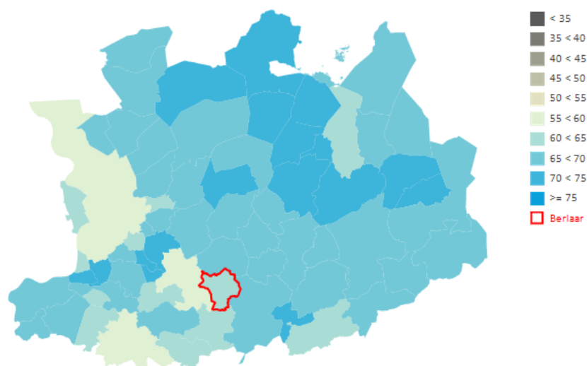
FIGUUR 1: Totale dekkingsgraad (%) per gemeente. Antwerpen 2015, 56-74 jarige mannen en vrouwen.
