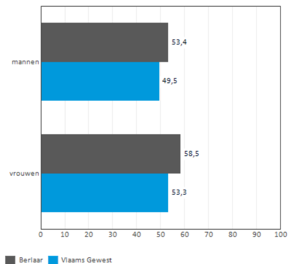
FIGUUR 6: Responsgraad (%) naar geslacht in 2015.
