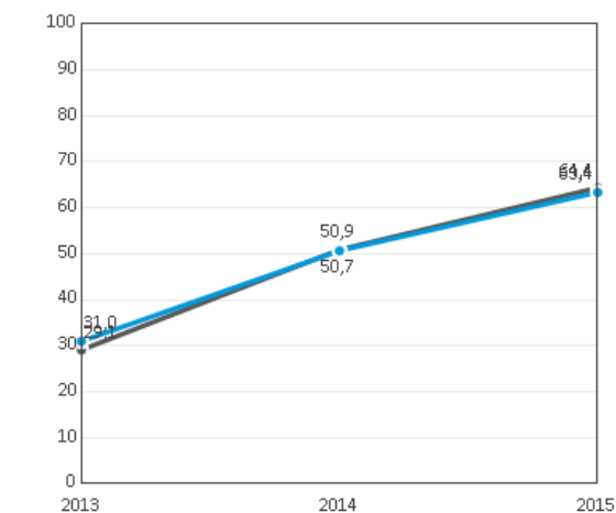
FIGUUR 7: Totale dekkinggraad (%) per jaar.
