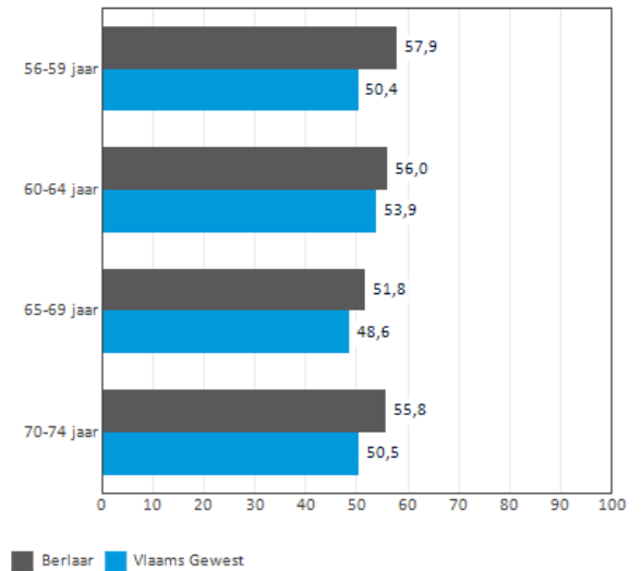
FIGUUR 4: Responsgraad (%) per 5-jarenklasse in 2015.
