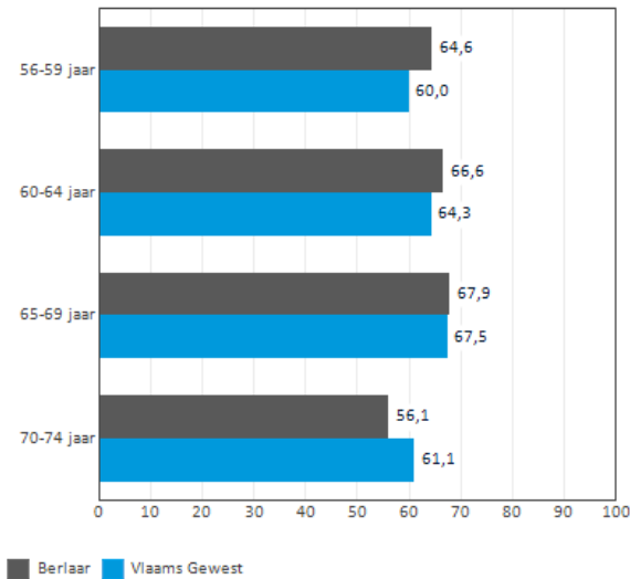
FIGUUR 3: Totale dekkinggraad (%) per 5-jarenklasse in 2015.
