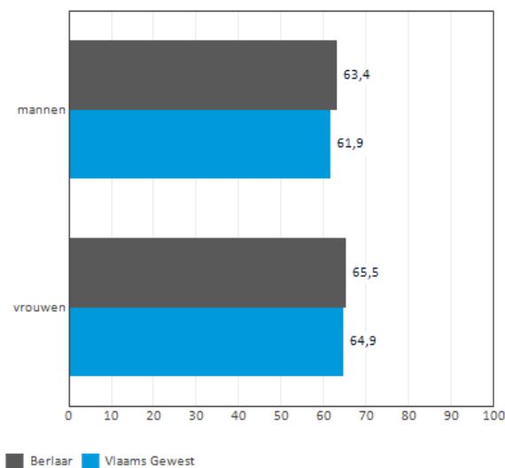
FIGUUR 5: Totale dekkinggraad (%) naar geslacht in 2015.
