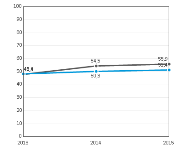
FIGUUR 8: Responsgraad (%) per jaar.
